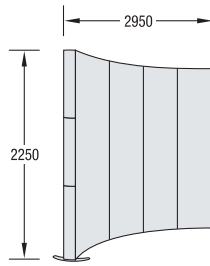
VA 5843 P1 für 4 Panels seitliche Aluminiumprofile silber eloxiert, inkl. 2 Spots
